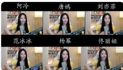
换 脸 软 件.
